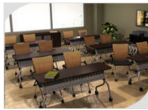
Sync Tables
